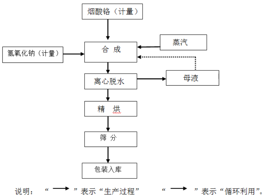
图 2-4 烟酸铬生产工艺流程图
