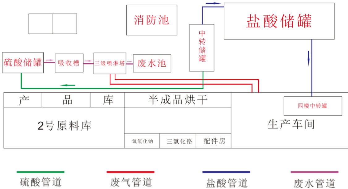
图 3-3 厂区管网图
