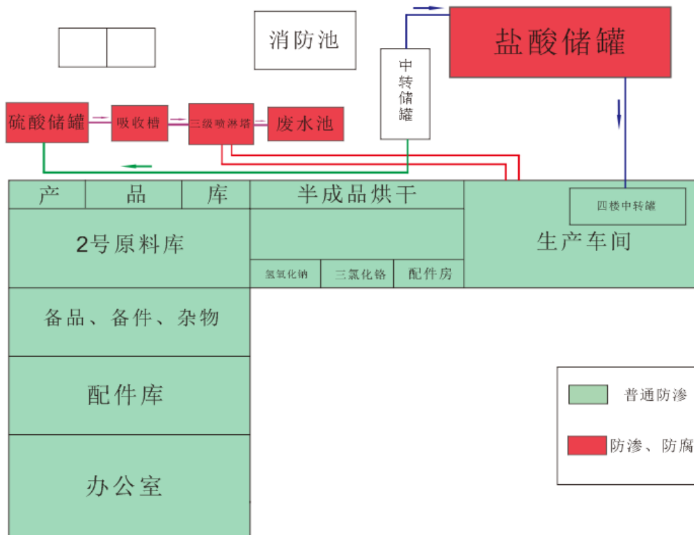
图 3-4 厂区防渗布置图
